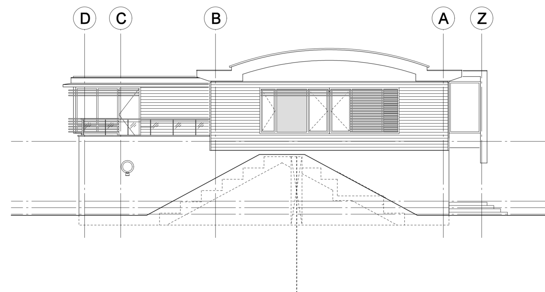
WESTGEVEL
