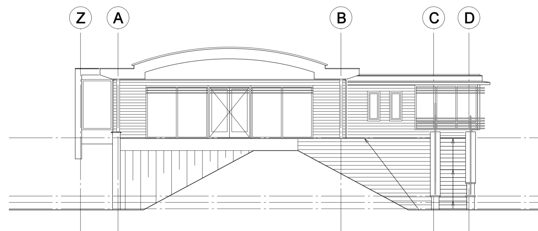
OOSTGEVEL
